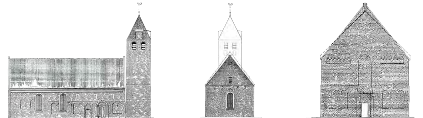
Tekeningen uit 1921 van G. Veenstra: Noordgevel
